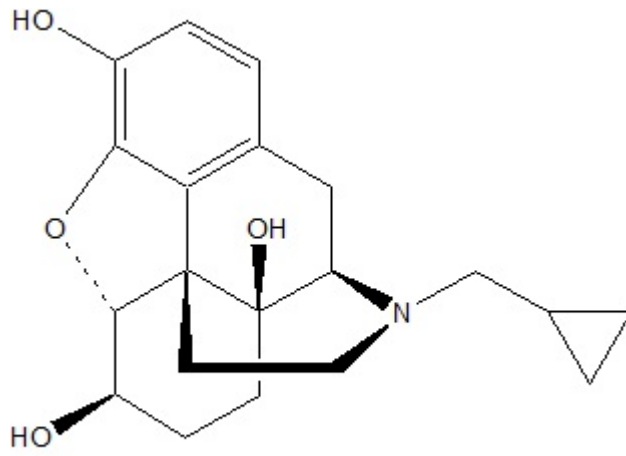
6beta-Naltrexol
