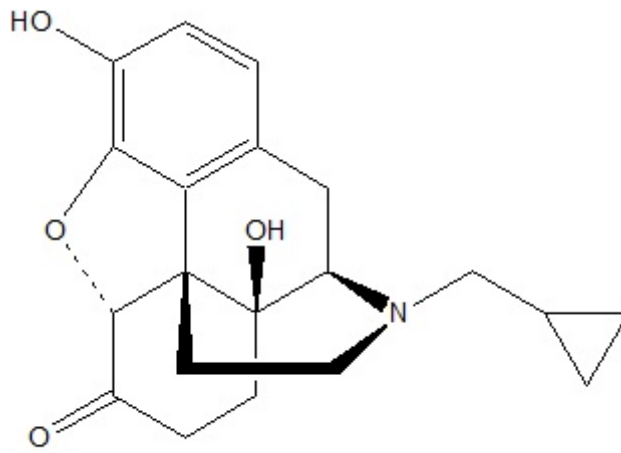
Naltrexone
